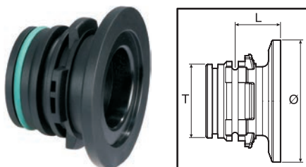
Adattatore flangiato tipo "Banjo" attacco maschio Flanged male connector "Banjo" type Adaptador embreado tipo "Banjo" empalme macho
